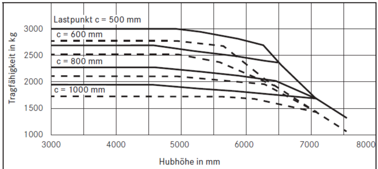
Tragfähigkeiten RX 60-30 mit Dreifach-Hubgerüst
